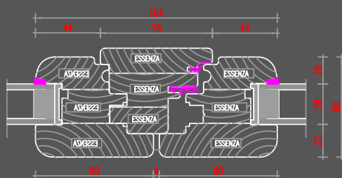
nodo centrale simmetrico
