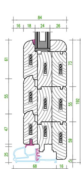
nodo inferiore portafinestra con vetro unico
