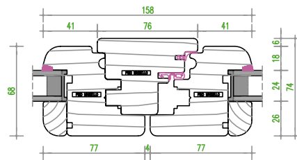
nodo centrale simmetrico
