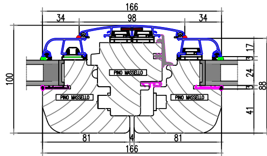
nodo centrale simmetrico
