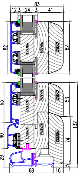
nodo inferiore portafinestra con traverso
