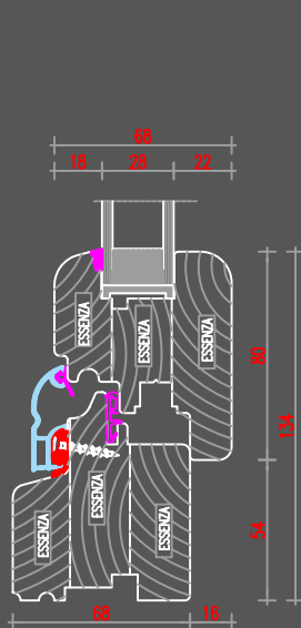
nodo inferiore finestra
