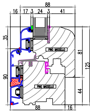
nodo inferiore finestra
