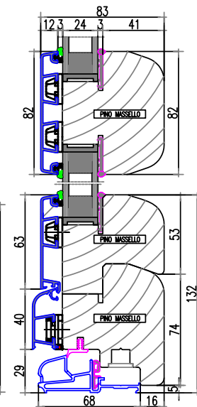
nodo inferiore portafinestra con traverso
