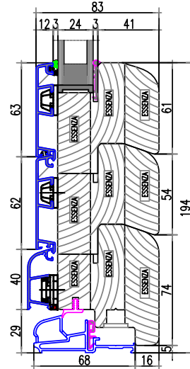
nodo inferiore portafinestra con vetro unico
