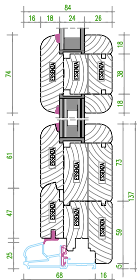
nodo inferiore portafinestra con trasverso
