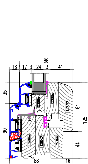
nodo inferiore finestra
