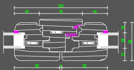
nodo centrale simmetrico
