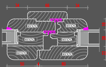
nodo centrale simmetrico
