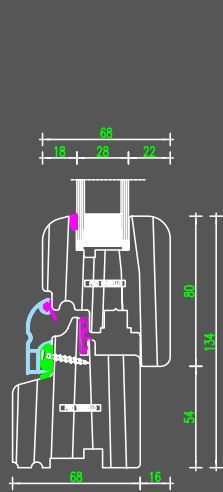
nodo inferiore finestra
