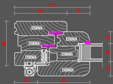
nodo centrale simmetrico
