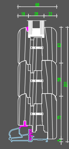
nodo inferiore portafinestra con vetro unico
