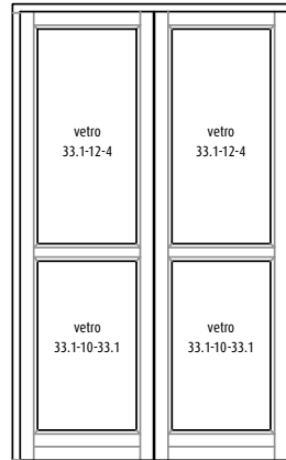
portafinestra con trasverso (PFT)
