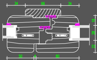
nodo centrale asimmetrico
