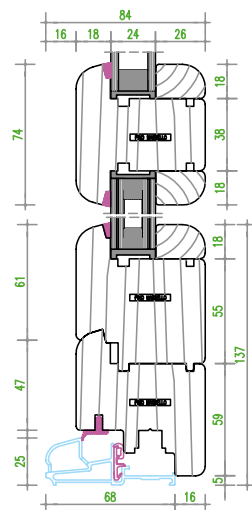
nodo inferiore portafinestra con traverso
