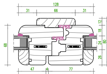
nodo centrale simmetrico
