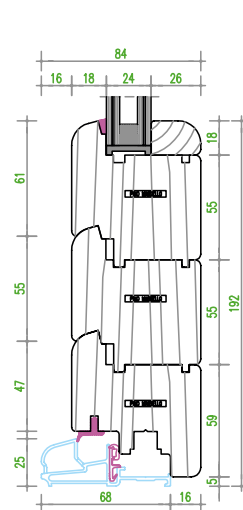
nodo inferiore portafinestra con vetro unico
