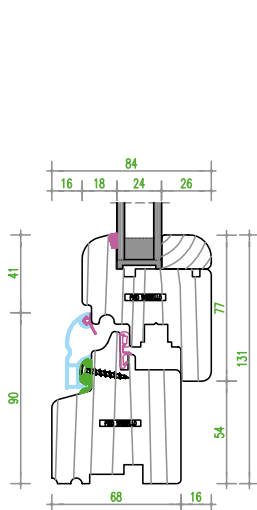
nodo inferiore finestra
