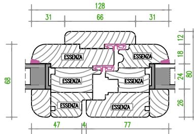
nodo centrale simmetrico
