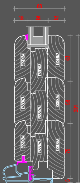
nodo inferiore portafinestra con traverso
