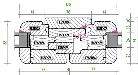
nodo centrale simmetrico
