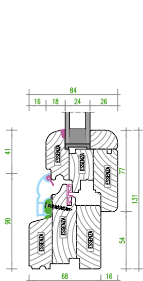
nodo inferiore finestra
